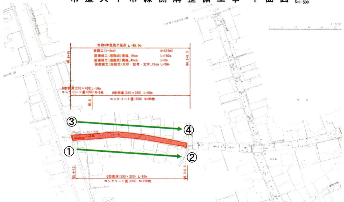
市道大下市線側溝整備工事 平面図 S=1:500
